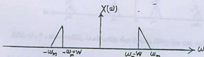
شکل ۱۰-۱۱. نمایش یک سیگنال میان گذر فرضی با نرخ نایکوئیست 2\omega_m و پهنای باند W
