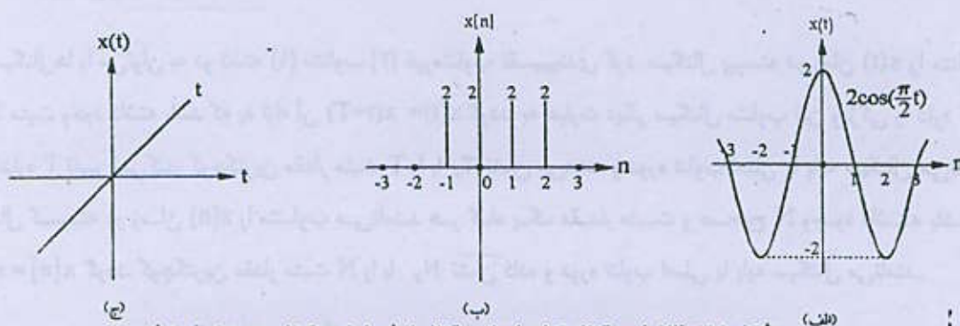
شکل ۱-۳. (الف) سیگنال توان (ب) سیگنال انرژی (ج) سیگنال غیر توان و انرژی
