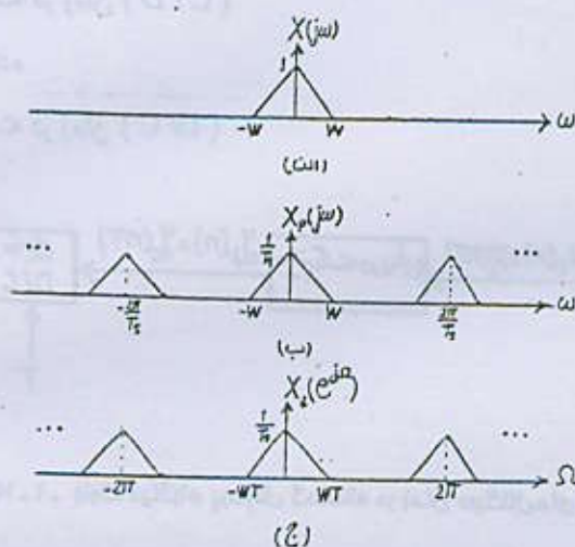
شکل ۱۶ - ۳ - طیف فرضی (الف) X(j\omega) (ب) X_p(j\omega) (ج) X_d(e^{j\Omega})
