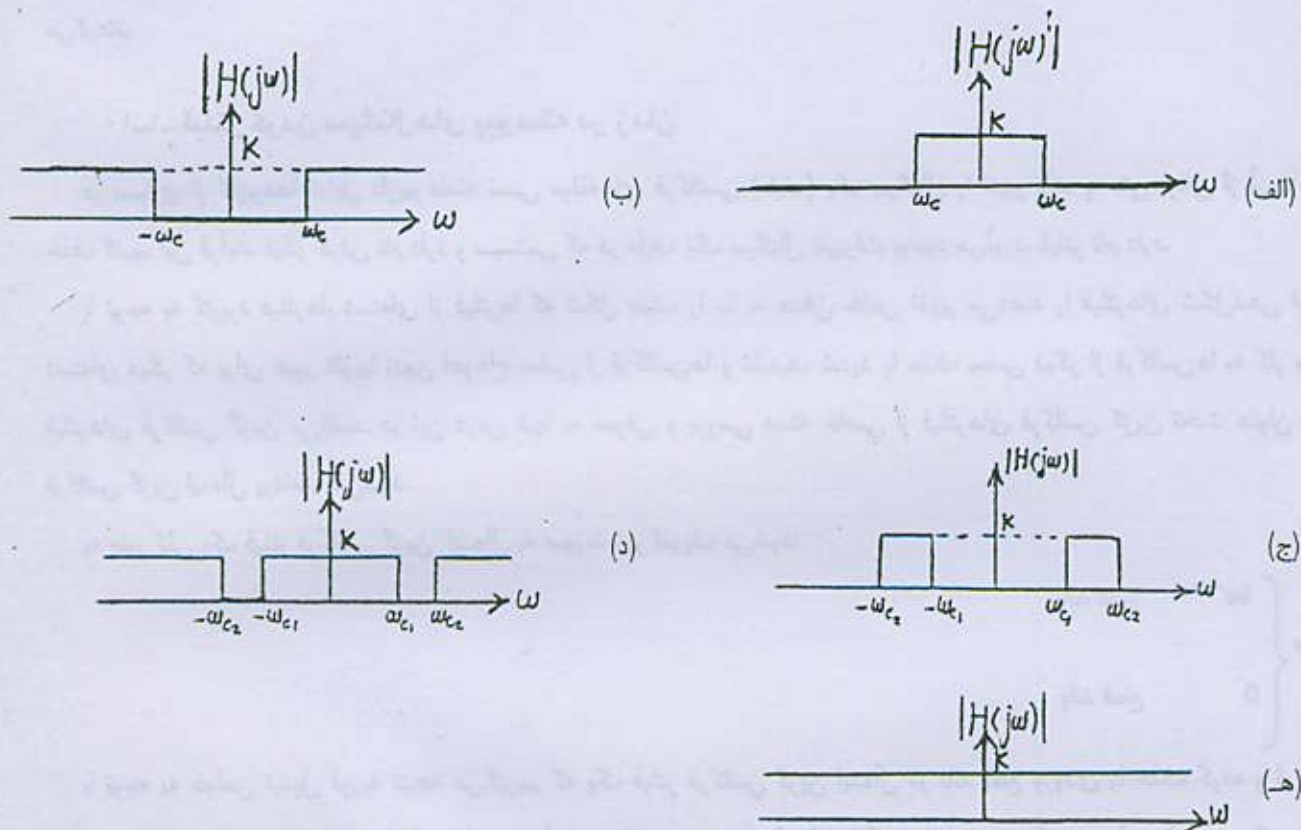
شکل ۱۰-۱-۱۰ پاسخ فرکانسی (الف) فیلتر پائین گذر ایده‌آل (ب) فیلتر بالاگذر ایده‌آل (ج) فیلتر
