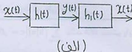
شکل ۵-۱. (الف) ترکیب سری یک سیستم وارون‌پذیر با سیستم وارون آن
