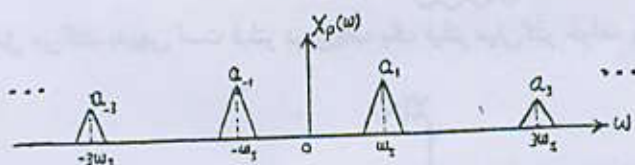
شکل ۹-۱۰ - طیف سیگنال نمونه‌برداری شده با فرض تقارن نیم موج سیگنال نمونه‌بردار
