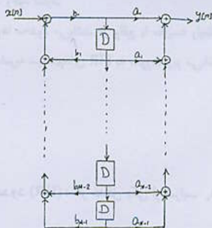
شکل ۴-۳. شکل کلی فرم مستقیم II
