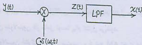
شکل ۱۵-۱۰-دمدولاتور DSB
