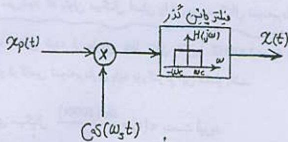
شکل ۱۰-۱۰. سیستم بازایی x(t) از x_p(t) برای حالتی که سیگنال نمونه بردار دارای تقارن نیم موج باشد.
