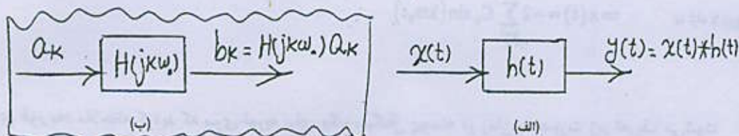
شکل ۸-۲. (الف) رابطه ورودی - خروجی یک سیستم LTI در حوزه (ب) رابطه بین ضرایب سری فوری ورودی و خروجی
