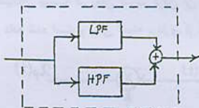
شکل ۳-۱۰. ترکیب موازی LPF و HPF که یک BPF را نتیجه می‌دهد
