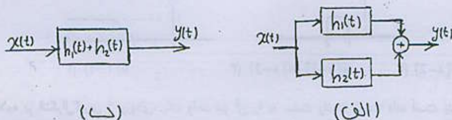
شکل ۴-۳ الف) ترکیب موازی دو سیستم LTI (ب) سیستم معادل ترکیب بند (الف)
