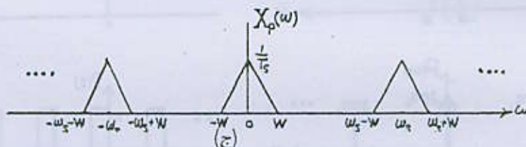
شکل ۱۰-۲. (الف) طیف فرضی برای x(t) (ب) طیف سیگنال نمونه برداری p(t) (ج) طیف سیگنال
