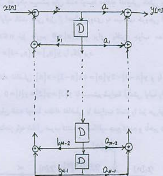
شکل ۶-۵ - شکل کلی فرم مستقیم II
