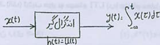
شکل ۳-۱۳. پاسخ ضربه انتگرال‌گیر برابر پله واحد است.
