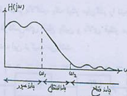
شکل ۵-۱۰. نمونه‌ای از پاسخ فرکانسی یک فیلتر پائین گذر غیر ایده‌آل
