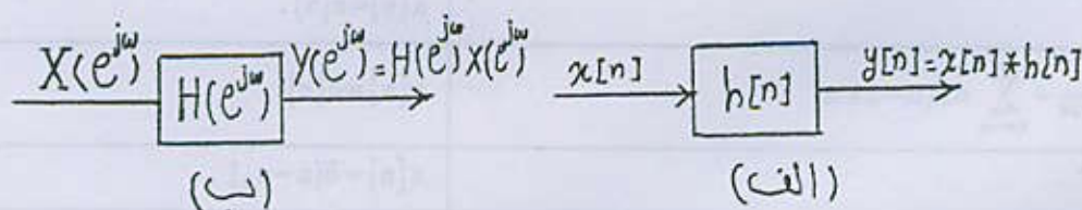
شکل ۱۳-۳. (الف) رابطه ورودی - خروجی یک سیستم LTI گسسته در حوزه (ب) رابطه بین تبدیل فوریه ورودی و خروجی
