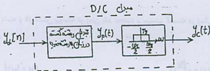
شکل ۱۴-۴. مبدل D/C
