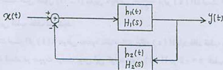
شکل ۱۷-۷ - اتصال فیدبک دو سیستم LTI
