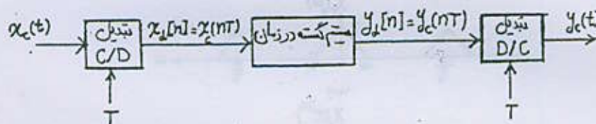
شکل ۱۶-۱. بلوک دیاگرام پردازش گسسته در زمان سیگنال‌های پیوسته در زمان
