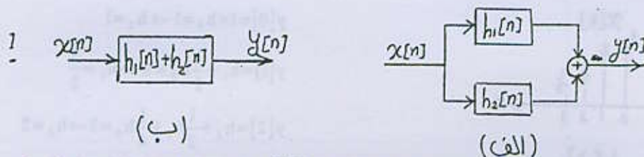
شکل ۴-۳. (الف) ترکیب موازی دو سیستم LTI (ب) سیستم معادل ترکیب بند (الف)
