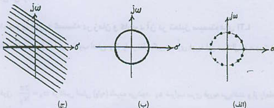
شکل ۱۱ - ۲ - مکان z ها در صفحه مختلط (الف) سری فوریه گسسته در زمان (ب) تبدیل فوریه گسسته در زمان (ج) تبدیل z
