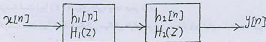
شکل ۱۸ - ۶. اتصال سری دو سیستم LTI گسسته
