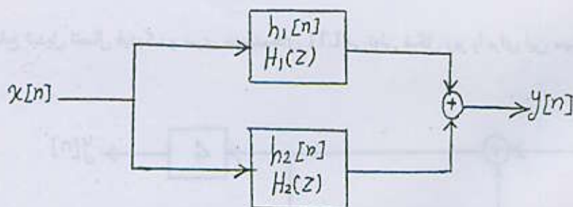
شکل ۱۸-۵ - اتصال موازی دو سیستم LTI گسسته
