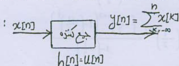
شکل ۴-۱. پاسخ ضربه جمع‌کننده برابر پله واحد است.
