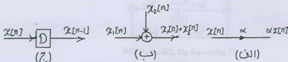
شکل ۴-۶. عناصر پایه جهت نمایش جعبه‌ای سیستم‌های گسسته در زمان توصیف شده توسط معادله تفاضلی خطی با ضرایب ثابت (الف) ضرب‌کننده در اسکالر (ب) جمع‌کننده (ج) تأخیر دهنده
