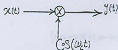
شکل ۱۰-۱۳. مدولاتور DSB
