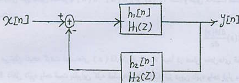
شکل ۱۸ - ۷. اتصال فیدبک دو سیستم LTI
