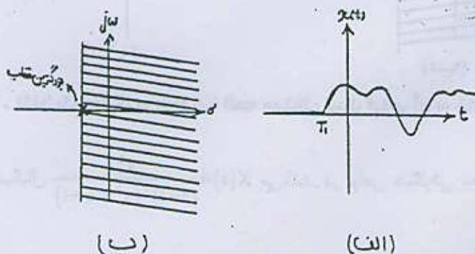
شکل ۱۷-۲. (الف) یک سیگنال سمت راستی (ب) نامیه همگرایی تبدیل لاپلاس آن به شکل \text{Re}\{s\} > \sigma_0
