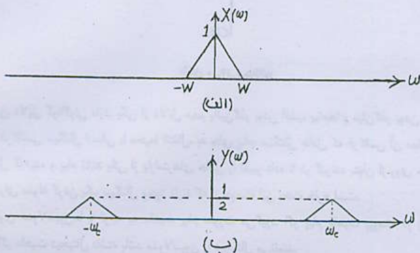
شکل ۱۴-۱۰-الف) طیف سیگنال پیام (ب) طیف سیگنال مدوله شده
