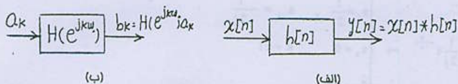
شکل ۱۲ - ۲ - (الف) رابطه ورودی - خروجی یک سیستم LTI گسسته در حوزه (زمان) (ب) رابطه بین ضرایب سری
