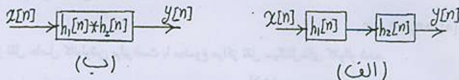
شکل ۳-۴. (الف) ترکیب سری دو سیستم LTI (ب) سیستم معادل ترکیب بند (الف)
