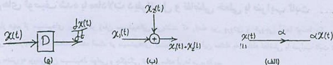
شکل ۴-۱. عناصر پایه جهت نمایش جعبه‌ای سیستم‌های پیوسته در (مان توصیف شده توسط معادله دیفرانسیل فطی با ضرایب ثابت
