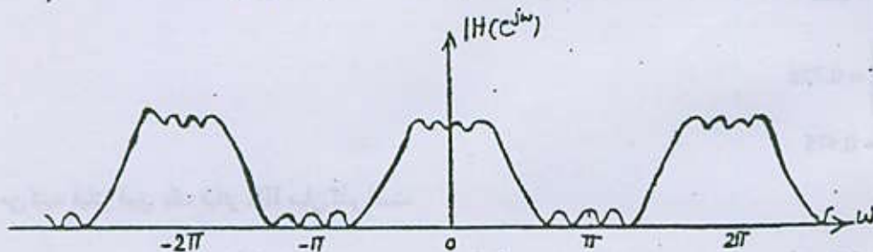
شکل ۱۴-۲ - نمونه‌ای از پاسخ فرکانسی یک فیلتر پائین‌گذر غیر ایده‌آل گسسته در زمان
