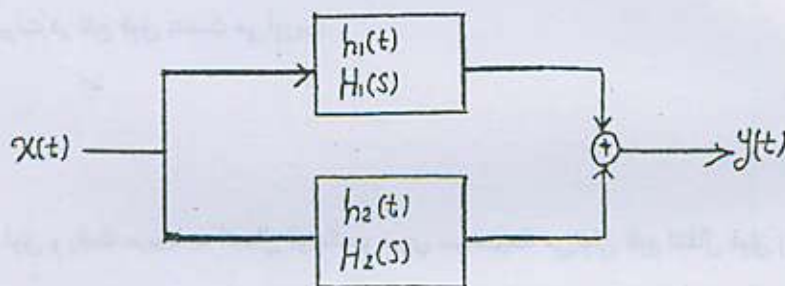
شکل ۱۷-۵ - اتصال موازی دو سیستم LTI
