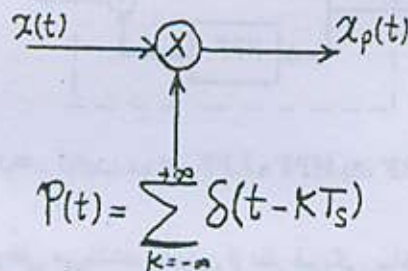
شکل ۵-۱۰. سیستم نمونه‌برداری ایده‌آل
