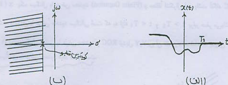
شکل ۱۷-۳. (الف) یک سیگنال سمت چپی (ب) نامیه همگرایی تبدیل لاپلاس آن به شکل \text{Re}\{s\} < \sigma_0
