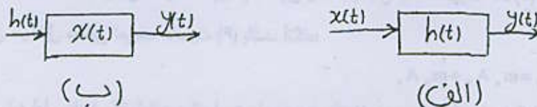
شکل ۳-۱۴. دو شکل نشان داده شده در (الف) و (ب) معادل می‌باشند.
