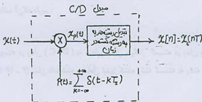
شکل ۱۶-۲. مبدل C/D
