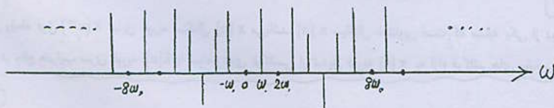
شکل ۱-۱۳- تبدیل فوری یک سیگنال گسسته متناوب فرضی با دوره تناوب N_0 = 8
