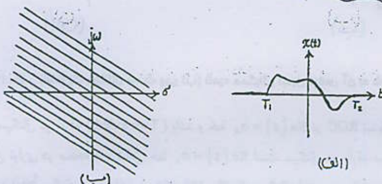
شکل ۱۷-۱. یک سیگنال با عرض محدود (ب) نامیه همگرایی تبدیل لاپلاس آن که کل صفحه s است.
