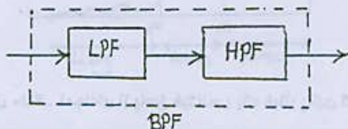
شکل ۳-۱۰. ترکیب سری LPF و HPF که یک BPF را نتیجه می‌دهد
