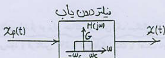
شکل ۱۰-۷. فیلتر پائین‌گذر ایده‌آل برای بازیابی x(t) از x_p(t)
