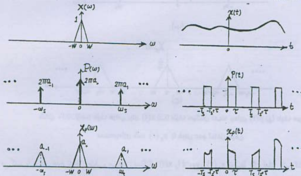
شکل ۸-۱۰. طیف و امپلیتود نمونه‌برداری غیر ایده‌آل توسط موج مربعی متناوب در موزه‌های زمان و فرکانس
