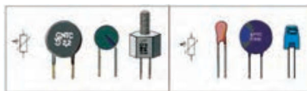
شکل ۱-۵۹- چند نمونه از مقاومت‌های P.T.C همراه با علامت فنی آن
