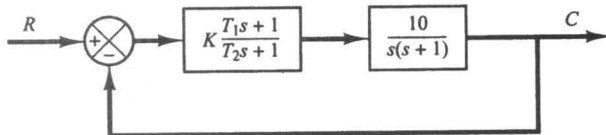
شکل ۶-۱۰۵ سیستم کنترل.
