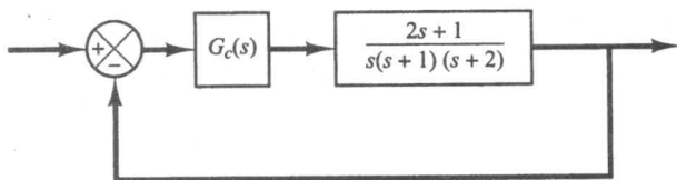
شکل ۶-۱۱۲ سیستم کنترل.
