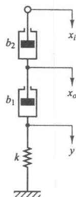
شکل ۶-۷۴ سیستم مکانیکی.
