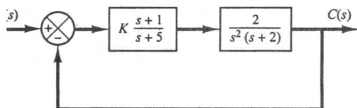
شکل ۱۰۰-۶ سیستم کنترل.
