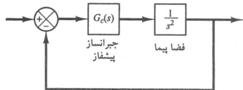
شکل ۱۰۸-۶ سیستم کنترل.
