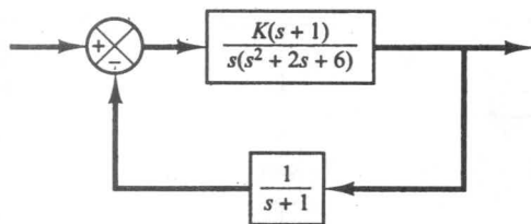
شکل ۱۰۱-۶ سیستم کنترل.
