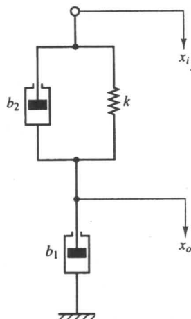
شکل ۶-۱۰۳ سیستم مکانیکی.
