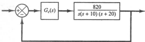
شکل ۱۱۰-۶ سیستم کنترل.
