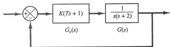
شکل ۶-۱۰۶ سیستم کنترل.
