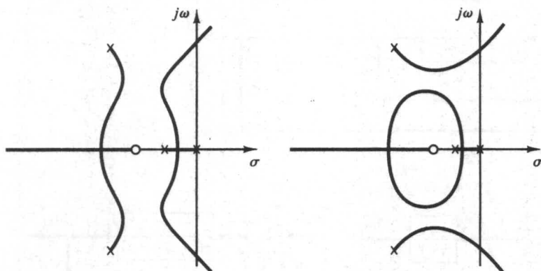
شکل ۱۳-۶ نمودارهای مکان هندسی ریشه‌ها.
