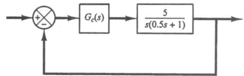
شکل ۱۰۷-۶ سیستم کنترل.
