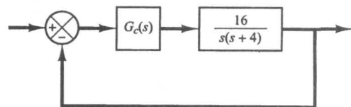
شکل ۱۰۹-۶ سیستم کنترل.
