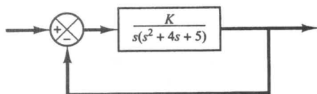
شکل ۶-۱۰۴ سیستم کنترل.
