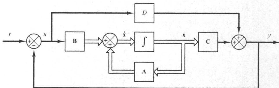
شکل ۱۹-۶ سیستم کنترل حلقه بسته.
