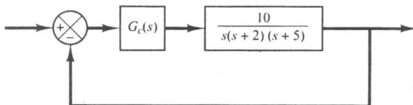
شکل ۱۱۱-۶ سیستم کنترل.
