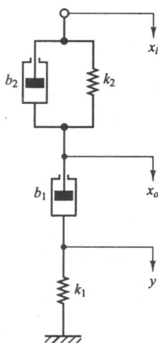
شکل ۷-۷۵ سیستم مکانیکی.
