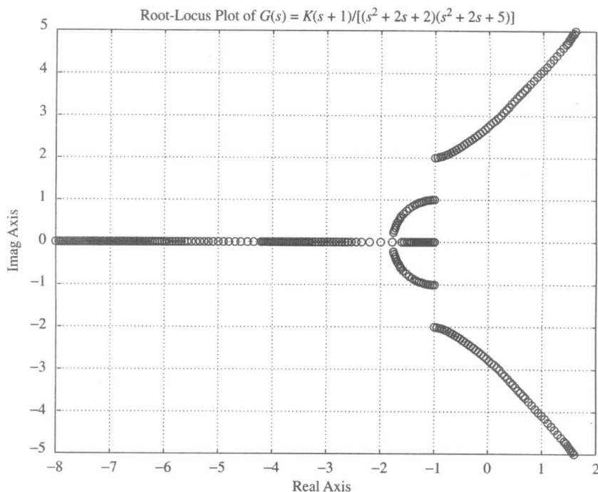
شکل ۶-۷۳ نمودار مکان هندسی ریشه‌ها.
