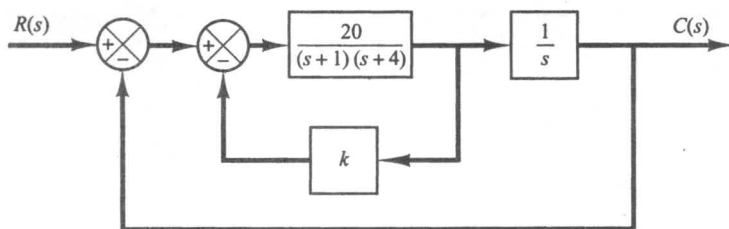
شکل ۶-۶۱ سیستم کنترل.
